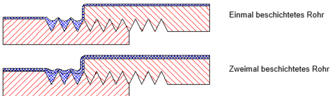
Abbildung 4: Verschraubung nach dem ersten und dem zweiten Beschichtungsschritt
